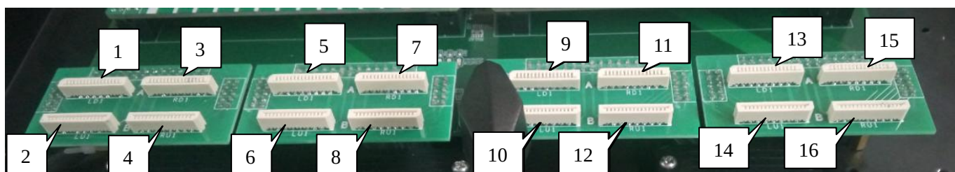
图 5.5 转接板数据线顺序图
