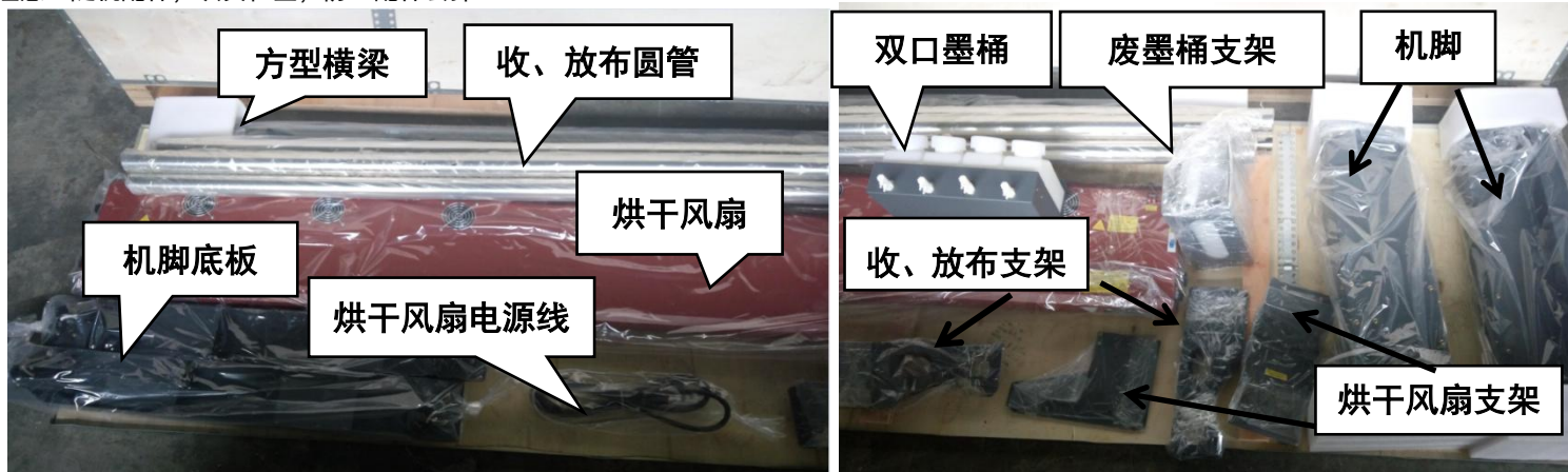
图 1.3 装机配件（一）图 1.4 装机配件（二）
