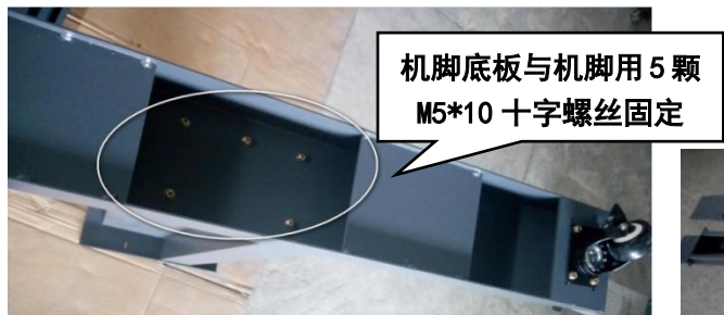
图 1.5 机脚与机脚底板安装示意图（一）
