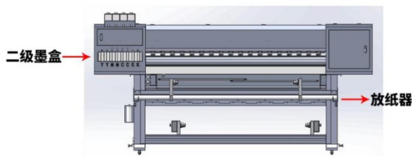
图 1.2 1.9-R 系列写真机图例（二）
