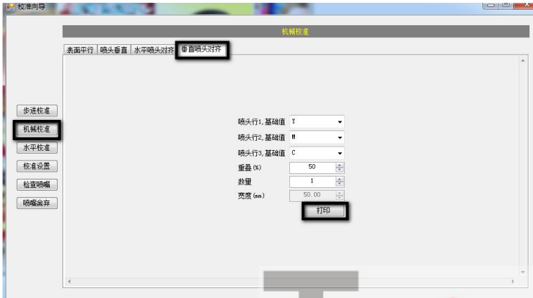
图 8.14 机械校准--垂直喷头对齐
