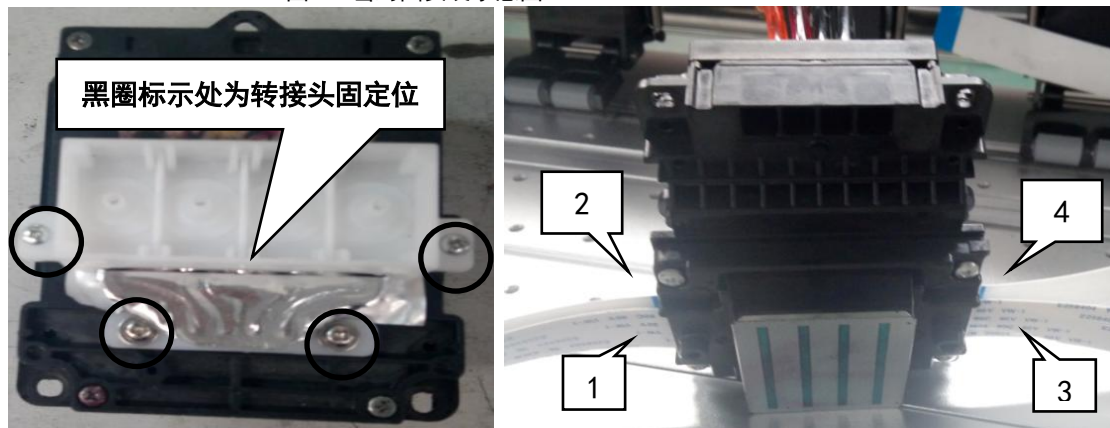
图 5.2 打印机喷头
