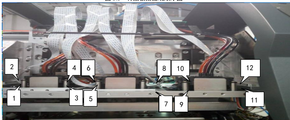
图 5.6 喷头数据线顺序图
