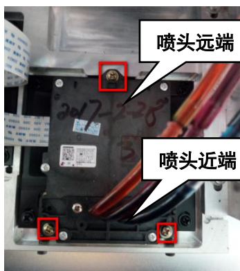
图 8.7.3 调整喷头机械位置
