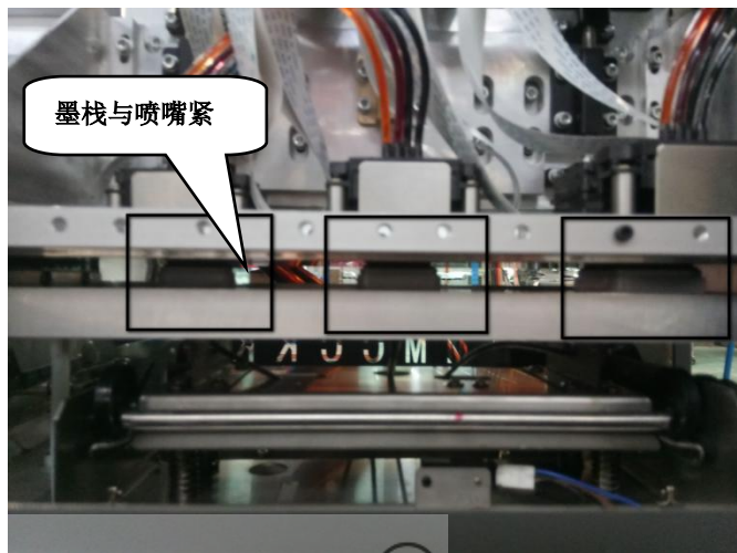
图 7.8 吸墨过程
