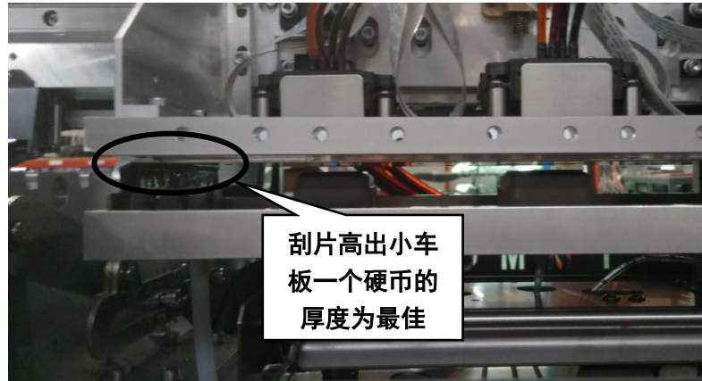
图 7.13 Z 移动过程
