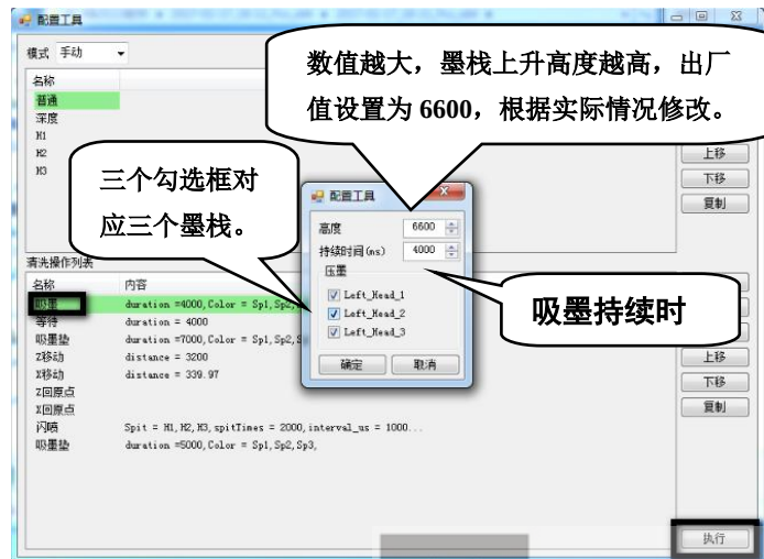
图 7.7 吸墨项内容
