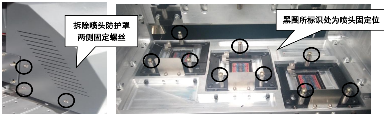
图 5.3 喷头固定位示意图
